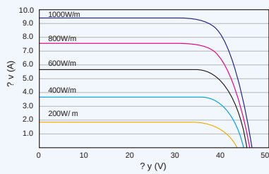
PVモジュール (335W) の I-V 曲線
