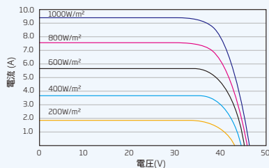
PVモジュール (335W) の I-V 曲線
